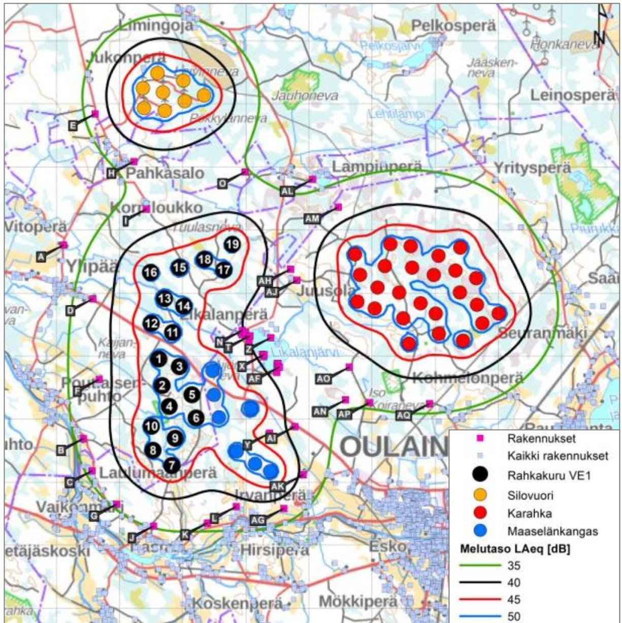
Kuva 35. Rahkakurun tuulipuiston melumallinnus VE1 -suunnitelma. (Lähde: Rahkakurun tuulivoimapaisto, Merijärvi, Suomi: Melu- ja väkelaskelmat. Kjeller Vindteknikk Oy, 2024)
